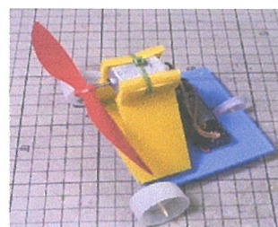
プロペラ車
