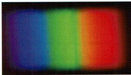
白熱灯の光
