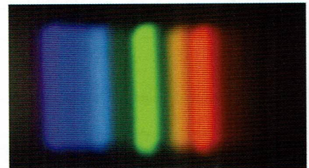
蛍光灯の光
